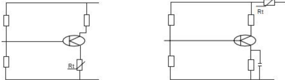
晶体管电路 transistor circuit
