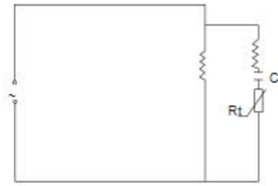
用于电容式电机电路 Capacitive motor circuit
