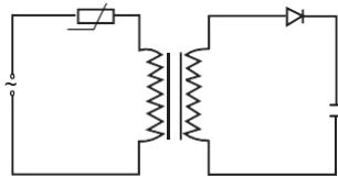
(a)用于电源变压器初级保护
